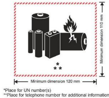
图 4: 锂电池标记
